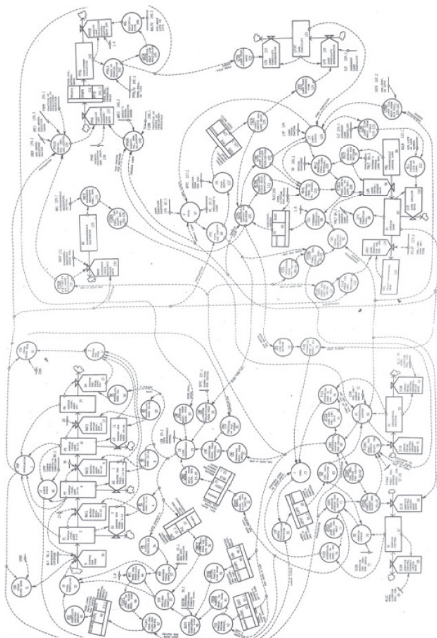
Figure 20 : Structure complète de World 3. Meadows et al. (1972a).
