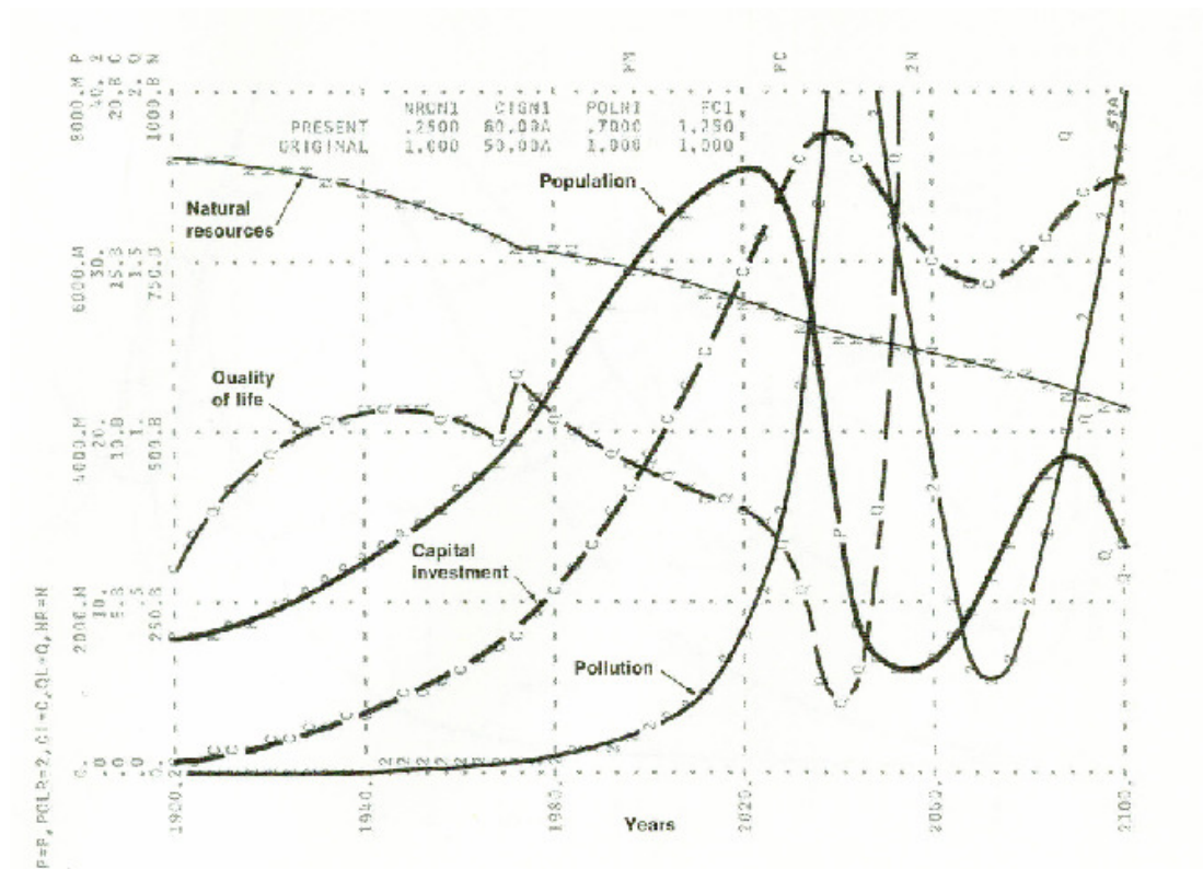
Figure 18 : Comportement désordonné de World 2 (hypothèses de production industrielle accrue). Forrester (1971), p.109.
