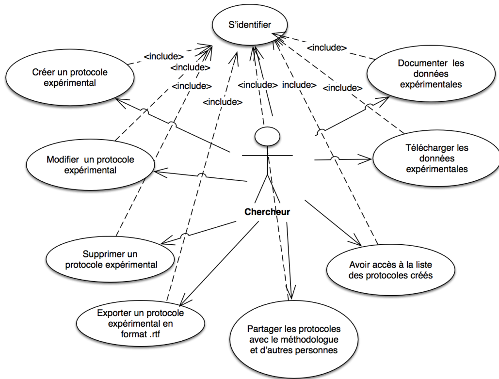
Figure 37 : Diagramme de cas d'utilisation de l'application pour le « Chercheur »
